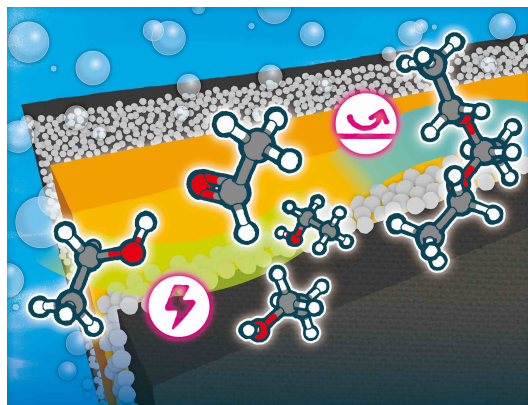
図1 電解デバイスによるエタノールからアセタールへの転換イメージ。電力を与えると分子の変換が進行する。
