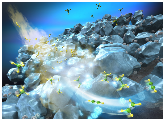
図2 メタンをカップリングして有用分子を合成するイメージ。難反応達成のためには触媒の高性能化が鍵を握る。
